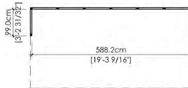
■ 3M X 6M PENISULA [penisula 10' x 20']
