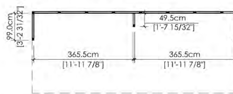
■ 3M X 7.5M INLINE [inline 10' x 24.5']
